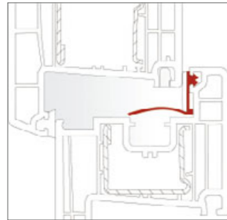
Lüfterstellung bei normalem Luftdruck
