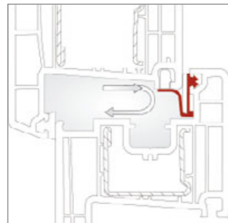
Bei steigendem Winddruck schließt der AirComfort automatisch nach dem Bernoulli-Prinzip
